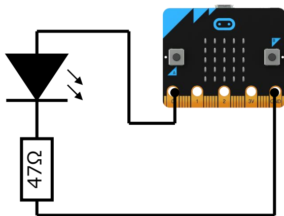
回路図
